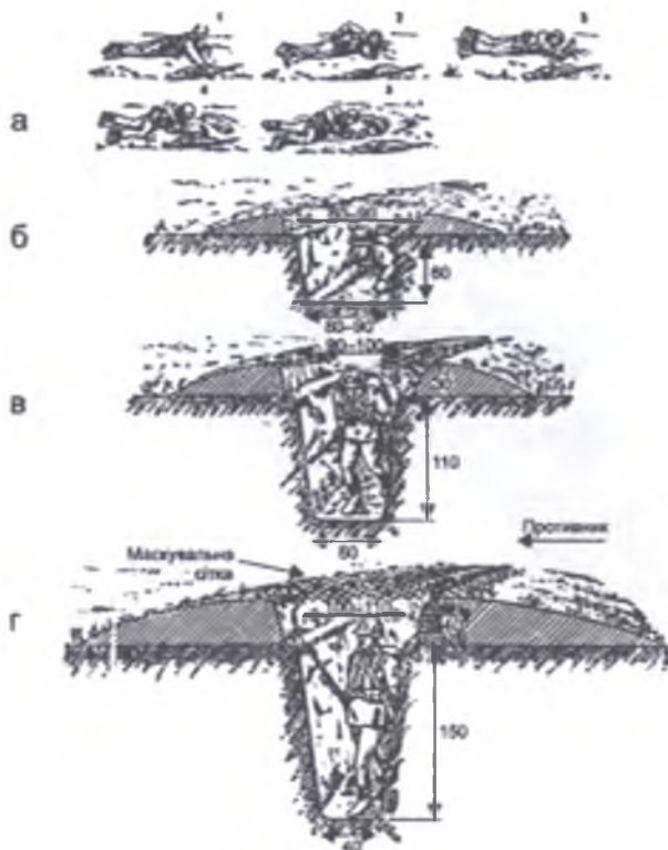
Ил. 7.4. Облаштування окопу солдатом у бойовій обстановці (усі розміри подані в см): а — послідовність роботи під час риття окопу для стрільби лежачи у випадку обстрілу противником; б — окоп для стрільби з коліна; в — окоп для стрільби стоячи; г — окоп для стрільби, замаскований маскувальною сіткою
