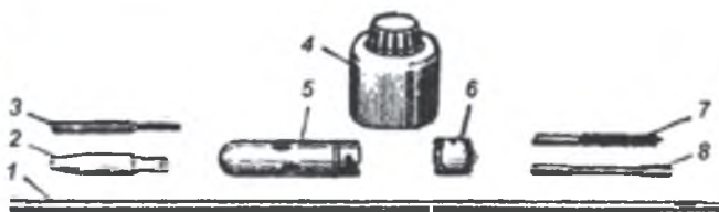
Іл. 13.5. а — місце для чищення автомата; б — приладдя для чищення автомата: 1 — шомпол; 2 — викрутка; 3 — вибивач; 4 — маслянка; 5 — корпус пенала; 6 — кришка пенала; 7 — кругла щітка; 8 — циліндрична протирка
