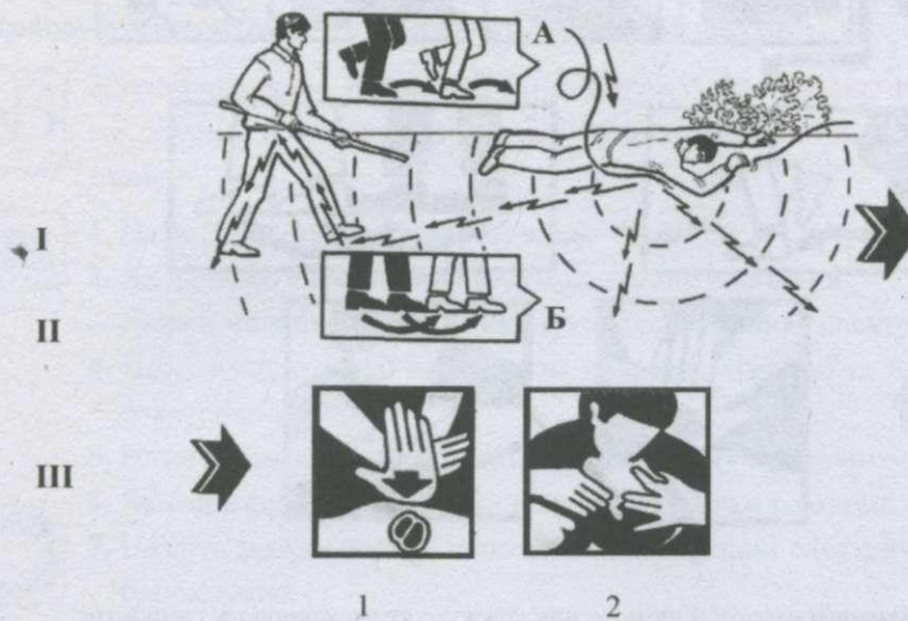
Іл. 8.1. Крокова напруга
