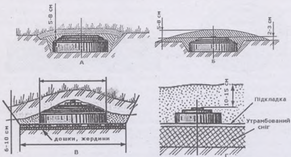
Іл. 10.2. Установлення протитанкової протиусясичної міни ТМ-57: А — у м'який ґрунт; Б — у твердий ґрунт; В — у заболочений ґрунт; Г — при глибокому сніжному покриві
