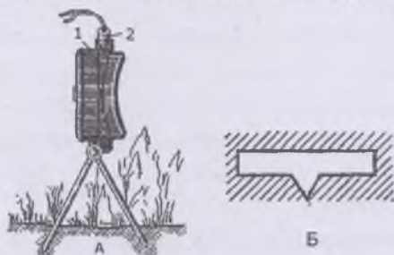
Іл. 10.8. А — встановлення міни МОН-50 з електродетонатором на ґрунт; 1 — корпус міни; 2 — пробка; Б — загальний вигляд прицільної щілини
