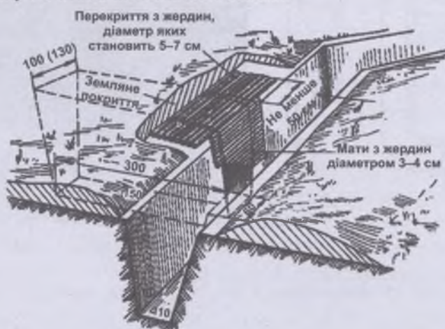
Іл. 16.2. Укриття для особового складу
